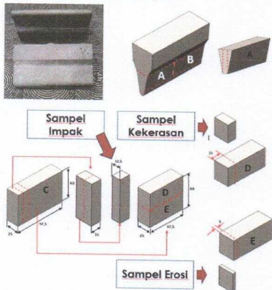
Gambar 2. Persiapan dan pemotongan material AISI 4140
