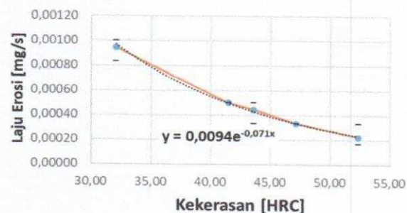
Gambar 5. Hubungan kekerasan dan laju erosi material AISI 4140 dari seluruh proses perlakuan panas
